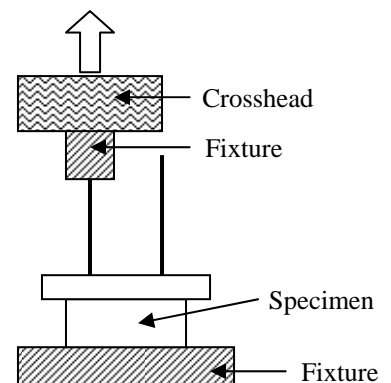
Figure 1 Tensile
